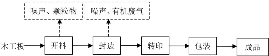
图 2 木门生产工艺流程图
