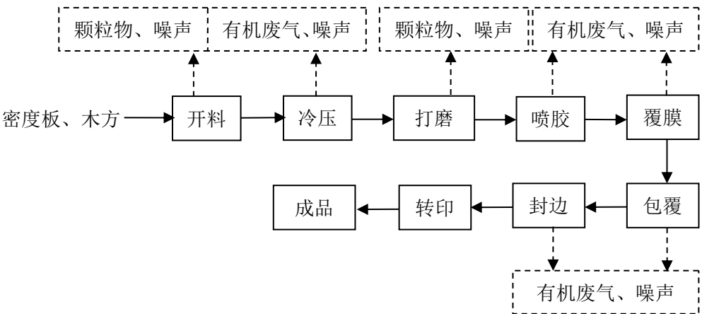
图 2 木门生产工艺流程图
