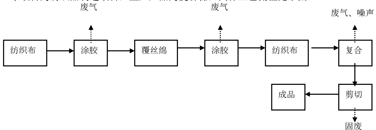
图2 复合棉生产工艺流程及主要污染情况图
