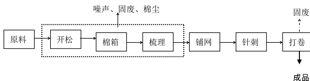
图 1 原有项目工艺流程图
