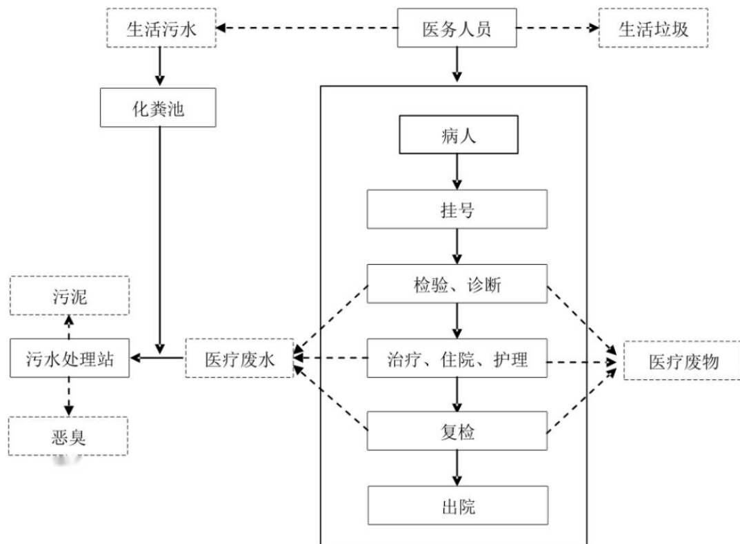
诊疗工艺流程及产污环节图
