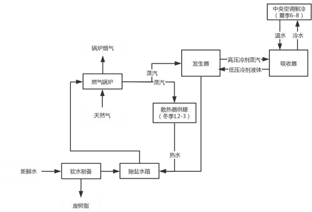
供暖、制冷工艺流程及产排污环节
