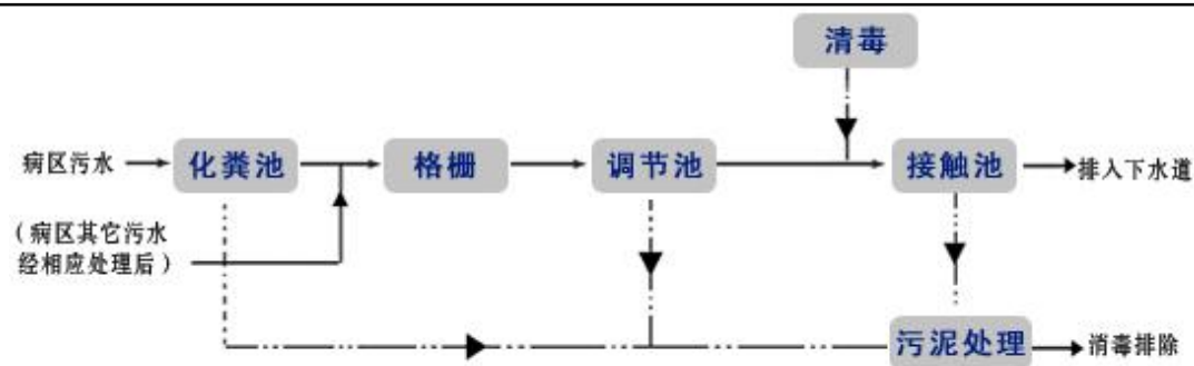
污水处理站处理工艺流程图
